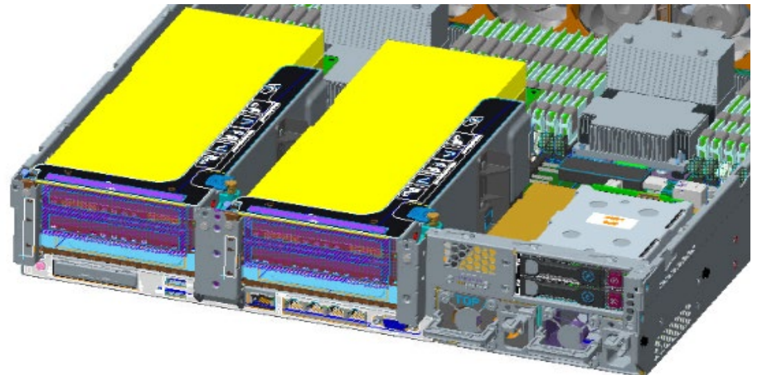
최대 2개 DoubleWide GPU 장착 + 디스크 2개 구성
