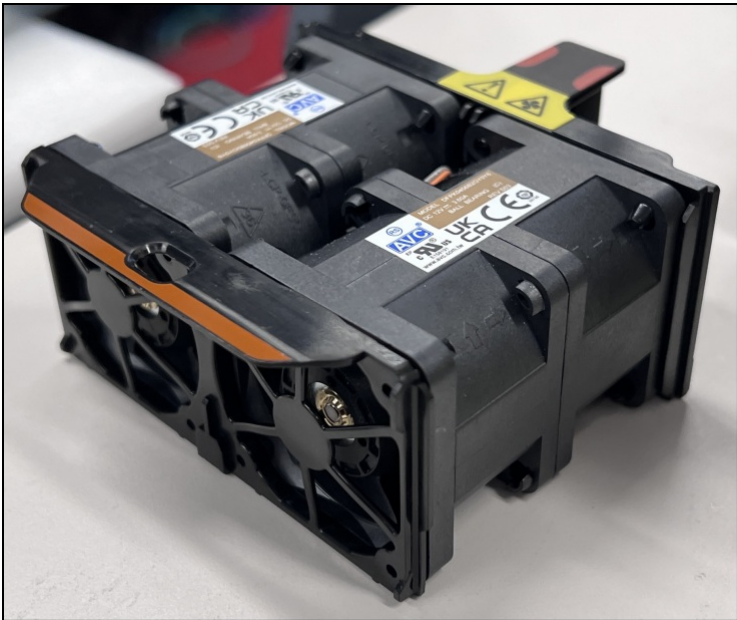
Figure 21. Fan module
