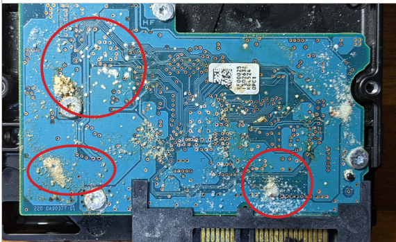
PCB 에 곰팡이가 있거나 녹이 슬거나 산화된 자국이 있음
