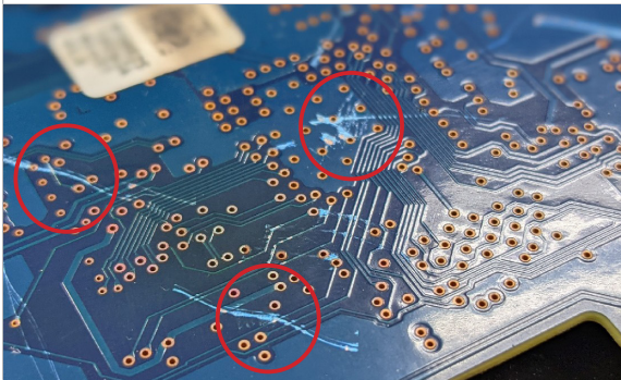
PCB 가 심하게 굽혀 회로가 손상됨
