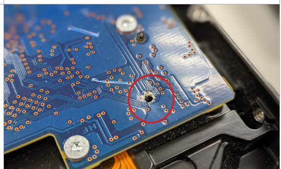
PCB 가 손상됨
