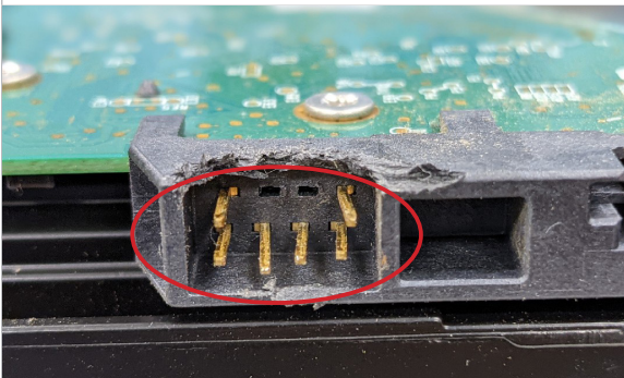
핀이 없음
