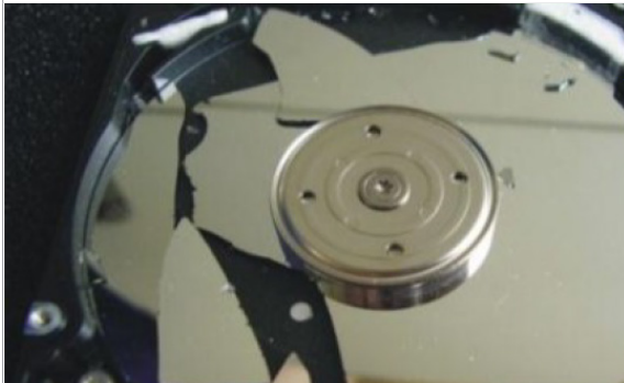
미디어가 손상됨 ( 드라이브가 기울어지면 손상된 미디어에서 소리가 남 )
