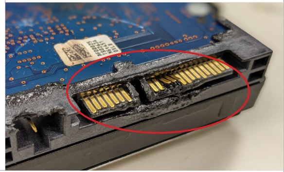
커넥터가 파손되거나 없음
