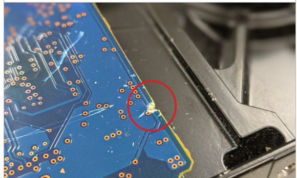
PCB 에 심하게 패인 자국이 있음
