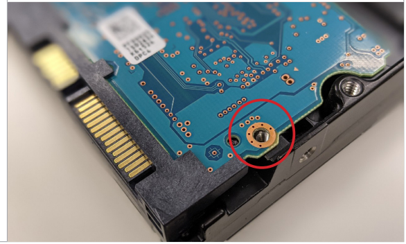
핀 가이드가 파손되거나 없음
