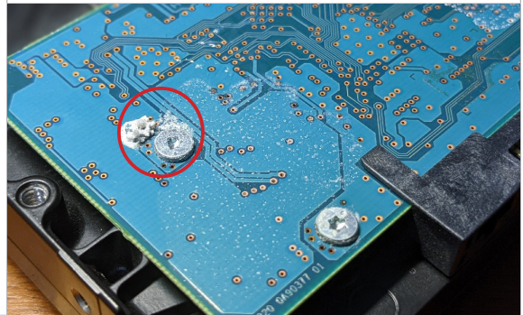
액체에 의해 손상됨
