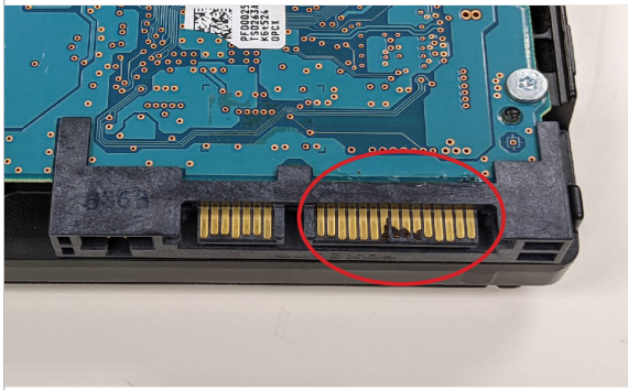
핀에 타거나 녹이 슬거나 산화된 자국이 있음
