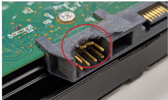
핀이 심하게 구부러짐
